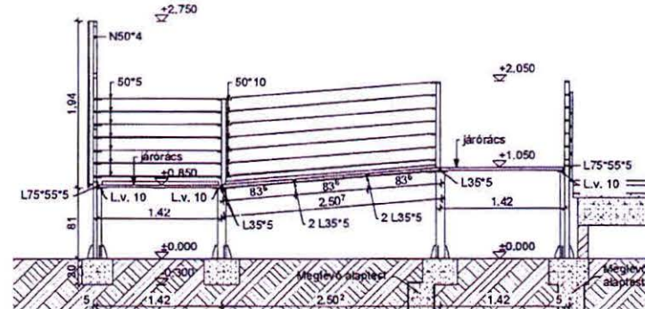
C-C METSZET
