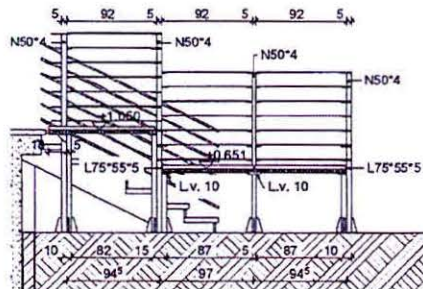
D-D METSZET
