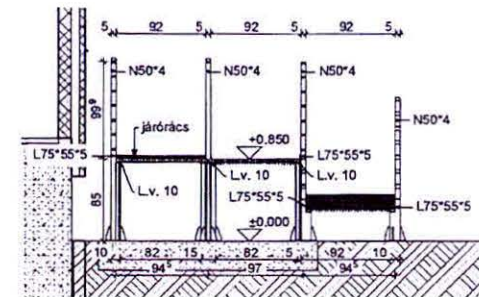
F-F METSZET
