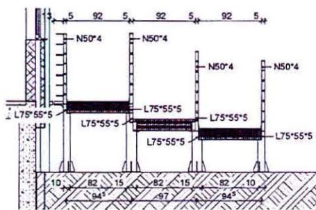
A-A METSZET
