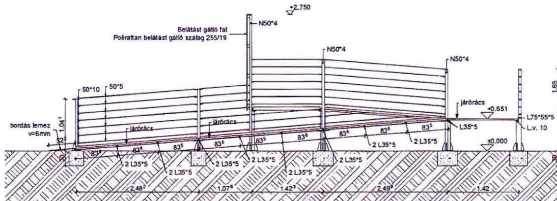
A-A METSZET
