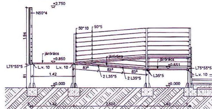
B-B METSZET
