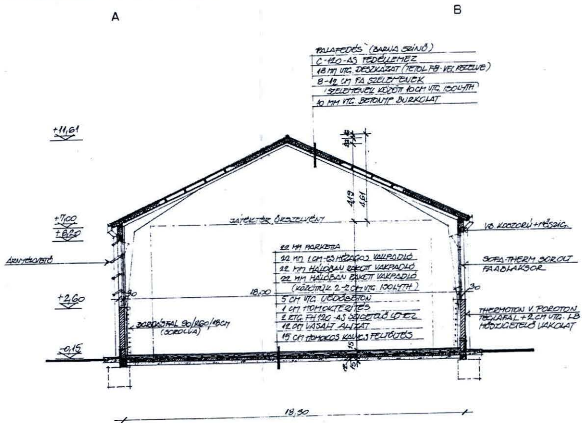
A-A METSZET
